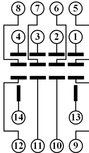
[ 14P 릴레이 소켓(DRS-09-14P) ]
