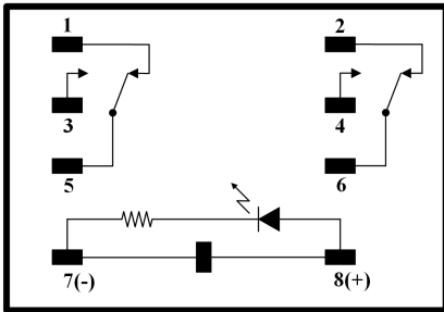
[ 8P 릴레이(CPBR용) ]
