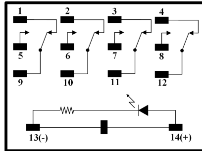
[ 14P 릴레이 (NPR, RPR, NWR, RWR용) ]
