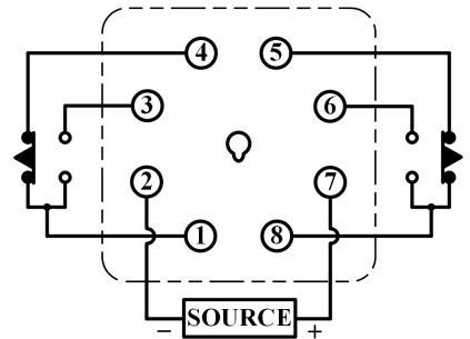
[ 8P 타이머릴레이 (T1용) ]
