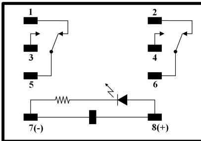
[ 8P 릴레이(RL용) ]
