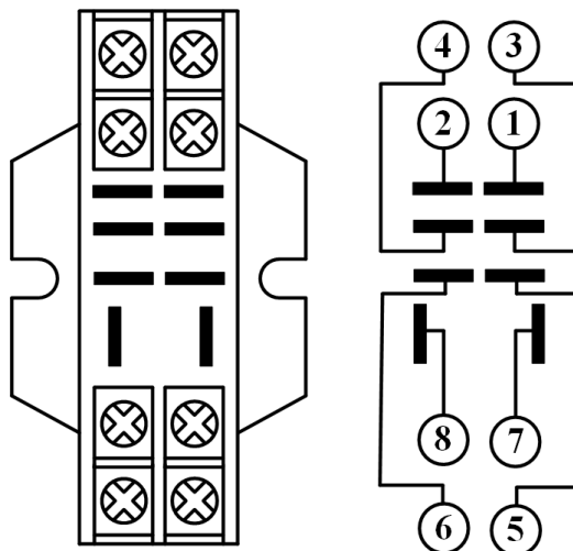
[ 8P 릴레이 소켓(DRS-04-8P) ]
