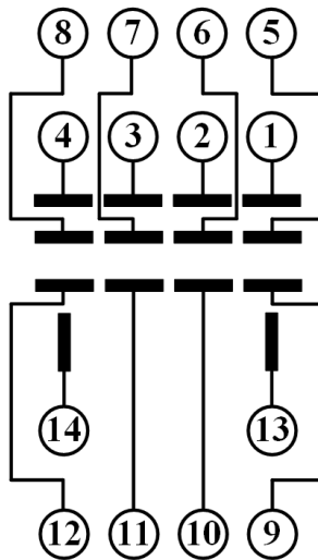
[ 14P 릴레이 (SR1, SR2, SPR1, SPR2용) ]
