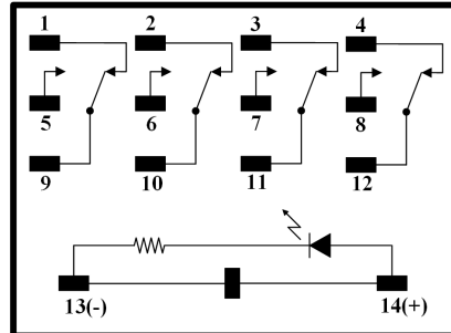
[ 14P 릴레이 (SR1, SR2, SPR1, SPR2용) ]
