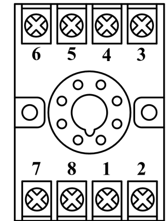
[ 8P 타이머릴레이 소켓 (PS-08) ]
