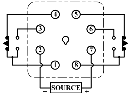
[ 8P 타이머릴레이 (STR용) ]
