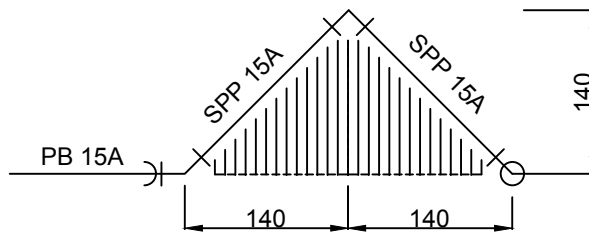
A - A' 단면도
