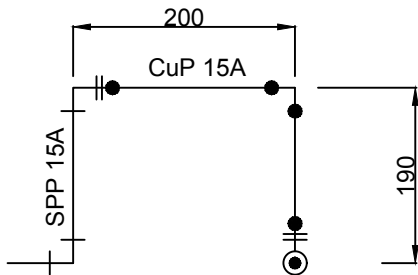
B - B' 단면도
