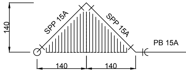
A - A' 단면도
