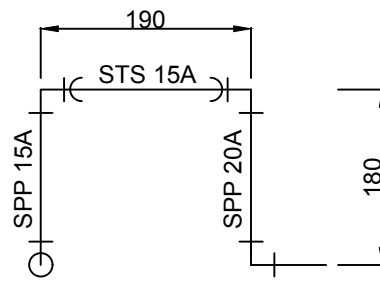
C - C' 단면도
