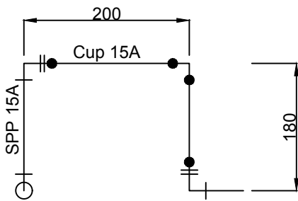
B - B' 단면도
