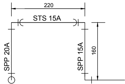
C - C' 단면도
