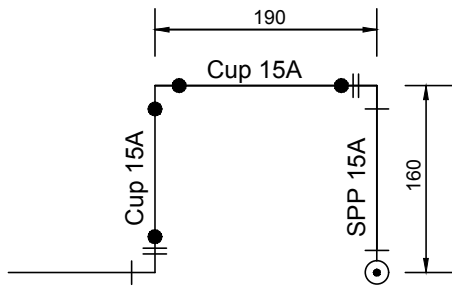
B - B' 단면도
